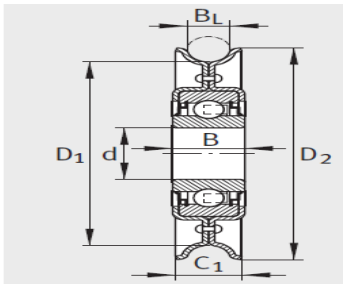
RSRD...LO 类型 D
