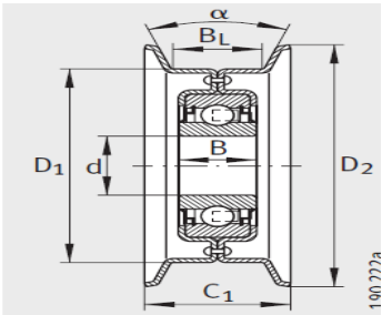
RSRB...LO 类型 B
