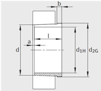
锥度为 1：12
