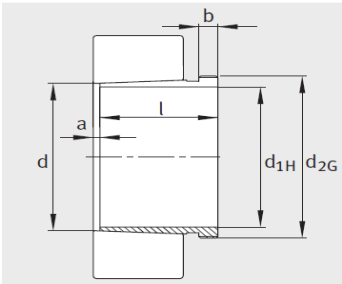
AH240、AH241 锥度为 1：30
