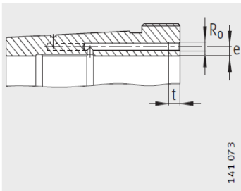
液压退卸套（后缀 H） 安装尺寸
