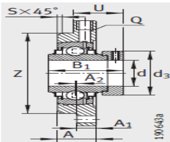
RMEO (从 d = 80 mm)
