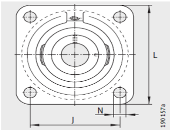
PCF、PCJ、PCJ...-FA125、RCJ、RCJ...-FA125、RCJ...-FA164、RCJO、TCJ、PCJY、RCJY、RCJY...-JIS、RCJL
